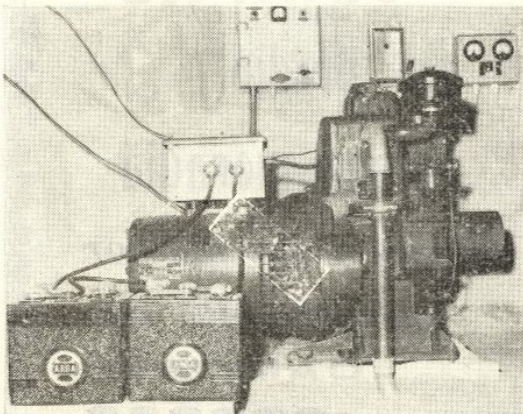
PORMENOR PARCIAL DUMA INSTALAÇÃO-TIPO
